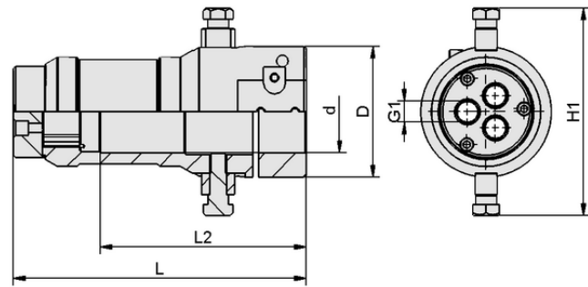
Tasarım verileri SXT-QC-CON-60-M-6
