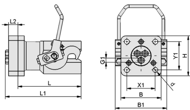
Données de construction SXT-QC-CON-40-F-3
