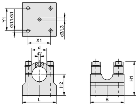
Dati di costruzione SXT-CL 60 AL
