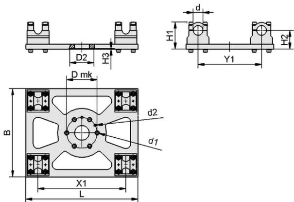
Données de construction SXT-RF-CL-D-160-40
