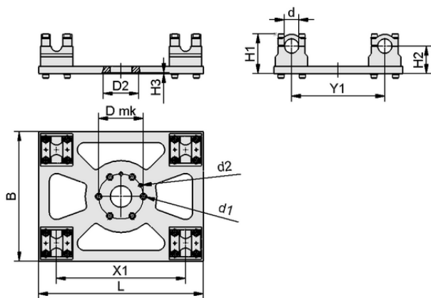
デザインデータ SXT-RF-CL-D-160-40
