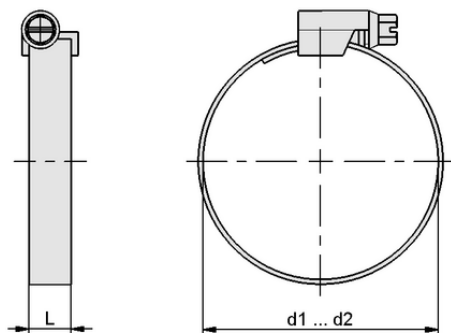
デザインデータ SSB 12-22 ST-VZ
