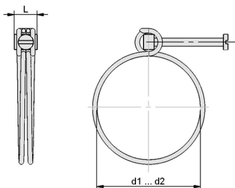
Données de construction SSD 35-40 ST-VZ
