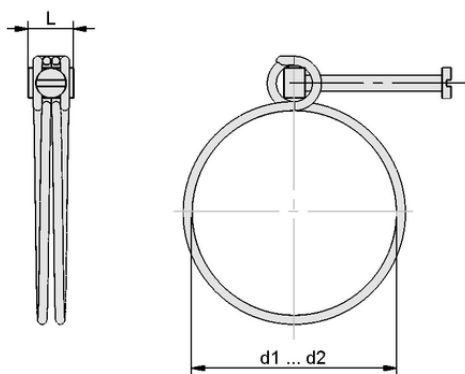
Données de construction SSD 60-68 ST-VZ
