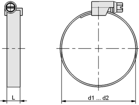
Tasarım verileri SSB 40-60 ST-VZ
