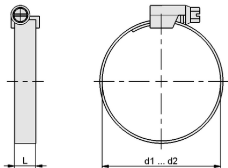
Datos de diseño SSB 32-50 ST-VZ
