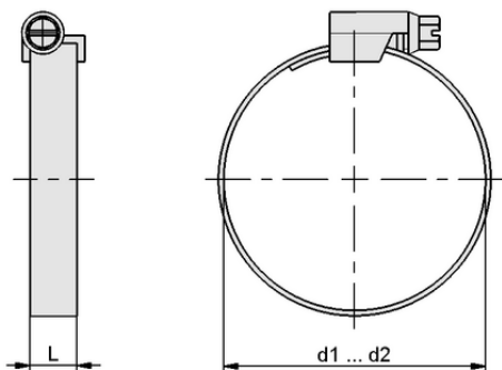
デザインデータ SSB 20-32 ST-VZ
