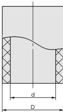
Konstruktionsdaten VSL 4-2.5 PU BL SO
