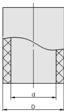
Données de construction VSL 6-4 PU BL SO
