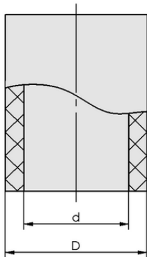
Datos de diseño VSL 6-4 PU BL SO
