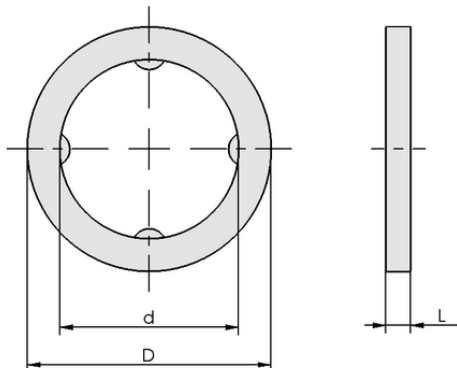
Données de construction DR G3/8 PA Easy-Fix
