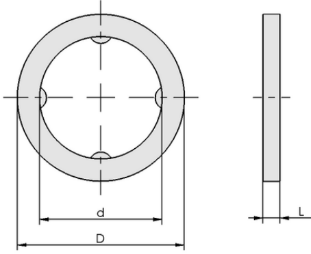
Tasarım verileri DR G1/8 PA Easy-Fix
