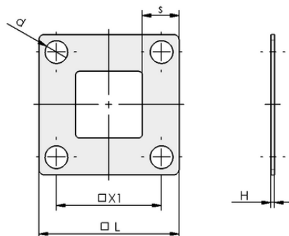
Datos de diseño DI-RA 40 PPTA MO-PROF
