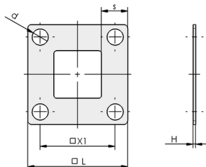
Konstruktionsdaten DI-RA 40 PPTA MO-PROF
