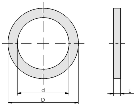
デザインデータ DR G1-1/4 49/42x2 PA
