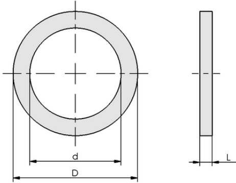
Tasarım verileri DR G1 39/34x2 PA
