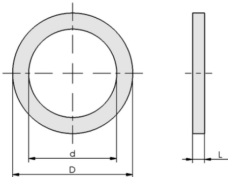
デザインデータ DR G3/4 33/27x2 PA
