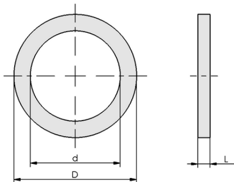
デザインデータ DR G1/4 18/13.5x1.5 PA
