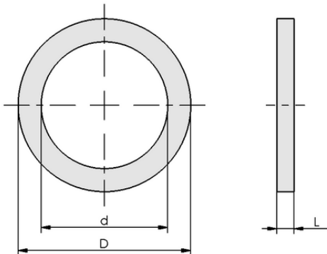
デザインデータ DR M5 8/5x1.2 PA
