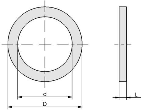
Tasarım verileri DR M5 8/5x1.2 PA
