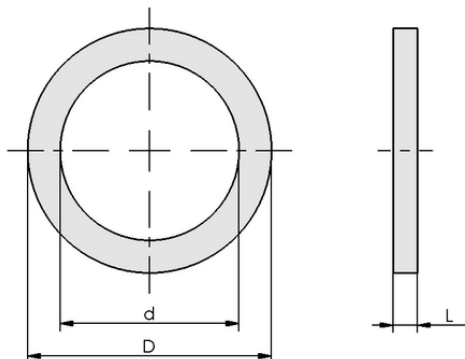
Données de construction DR M3 6/3.5x1 PA
