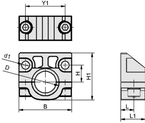
Tasarım verileri HP-HT 2M8 56 HT-A3
