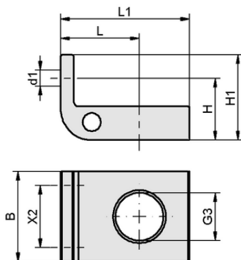
Dati di costruzione HP-FST 2M6 35 M20x1.5
