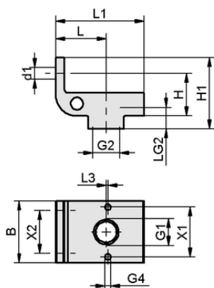
デザインデータ HP-SG 2M6 E 35 G3/8-IG
