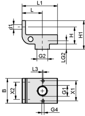
Tasarım verileri HP-SG 2M6 E 35 G1/4-IG
