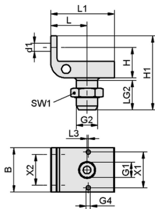
Design data HP-SG 2M6 E 35 G3/8-AG
