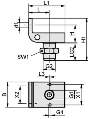
Tasarım verileri HP-SG 2M6 E 35 G3/8-AG
