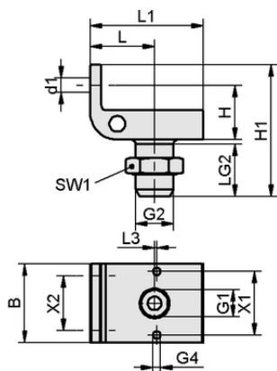
Dati di costruzione HP-SG 2M6 E 35 G1/4-AG
