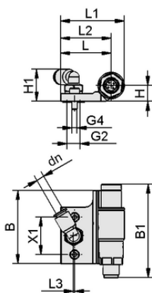
Dati di costruzione SET HT-SG..E VSi-HD M4x12
