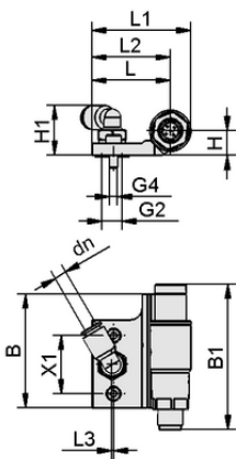
Konstruktionsdaten SET HT-SG..E VSi-HD M4x12
