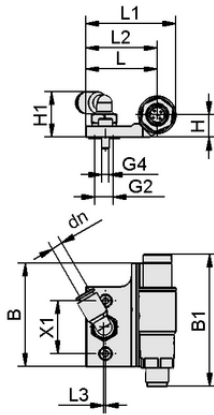
Tasarım verileri SET HT-SG..E VSi-HD M4x12
