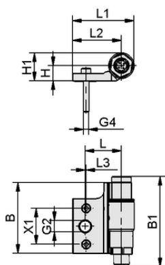
Dati di costruzione SET HT-SG..E VSi-HD M4x30
