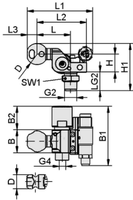
Tasarım verileri HT-SG A5 I 10 31 NPT3/8-AG AV VS
