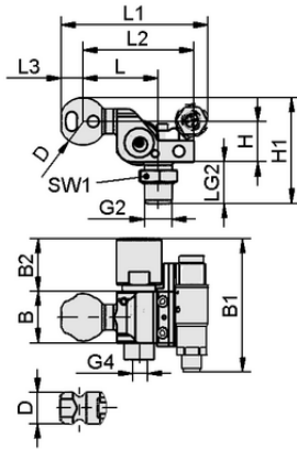
Tasarım verileri HT-SG A5 I 10 31 G3/8-AG AV VS
