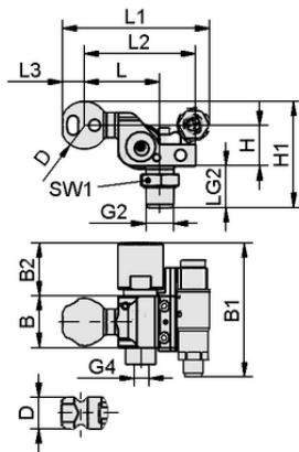
Dati di costruzione HT-SG A3 I 10 31 G3/8-AG AV VS
