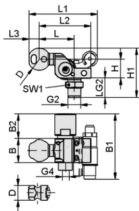
Dati di costruzione HT-SG A3 I 10 31 G3/8-AG AV
