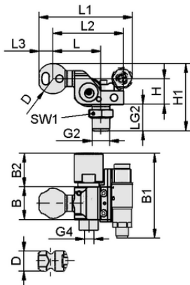
Design data HT-SG A2 I 10 31 NPT3/8-AG AV VS
