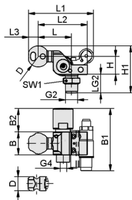
Dati di costruzione HT-SG A2 I 10 31 NPT3/8-AG AV
