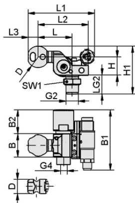
Design data HT-SG A2 I 10 31 G3/8-AG AV VS
