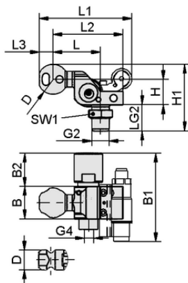
Design data HT-SG A2 I 10 31 G3/8-AG AV
