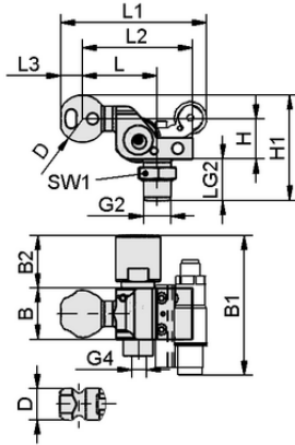
Tasarım verileri HT-SG A2 I 10 31 G3/8-AG AV
