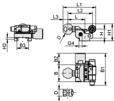
デザインデータ HT-SG A2 I 10 46 RA AV VS
