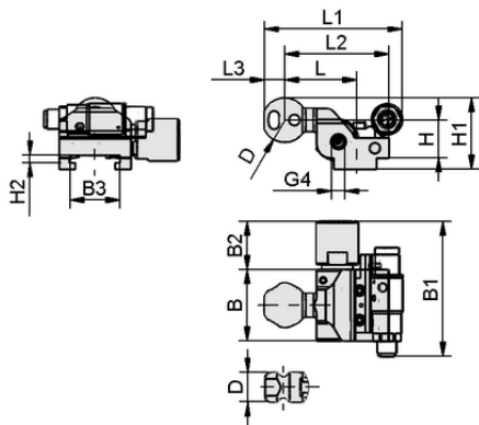
Design data HT-SG A2 I 10 46 RA AV VS
