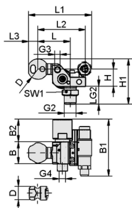
デザインデータ HT-SG A2 I 10 31 NPT3/8-AG AB VS
