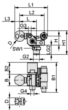
Konstruktionsdaten HT-SG A2 I 10 31 G3/8-AG AB VS
