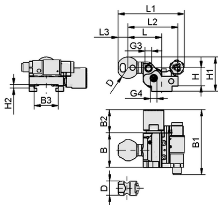
Design data HT-SG A3 I 10 46 RA AB VS
